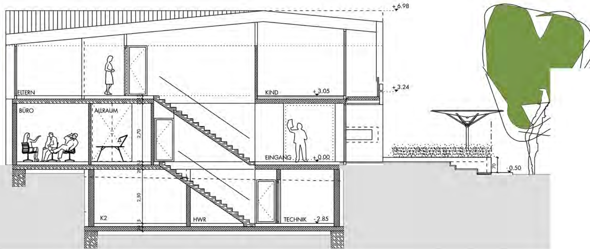
Schnitt 1-1
